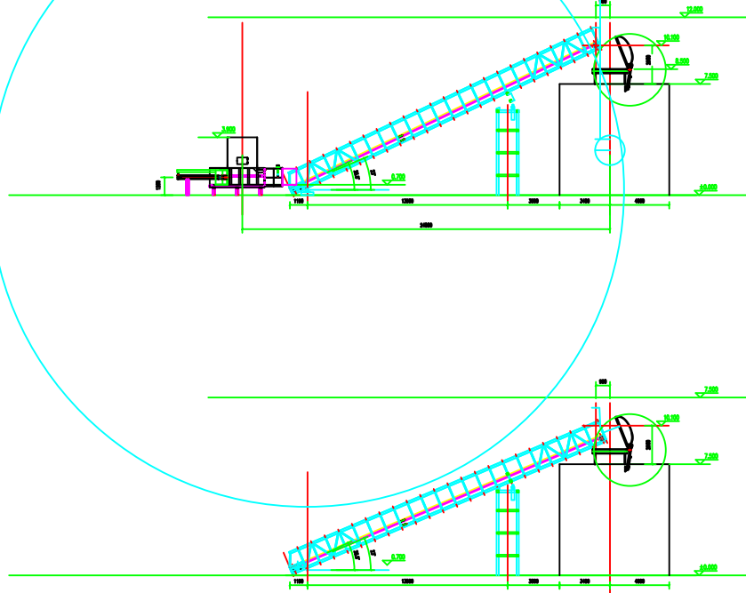
总装配图
